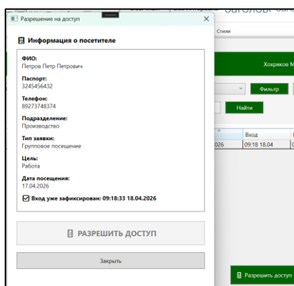
Рисунок 6 – Разрешение доступа
